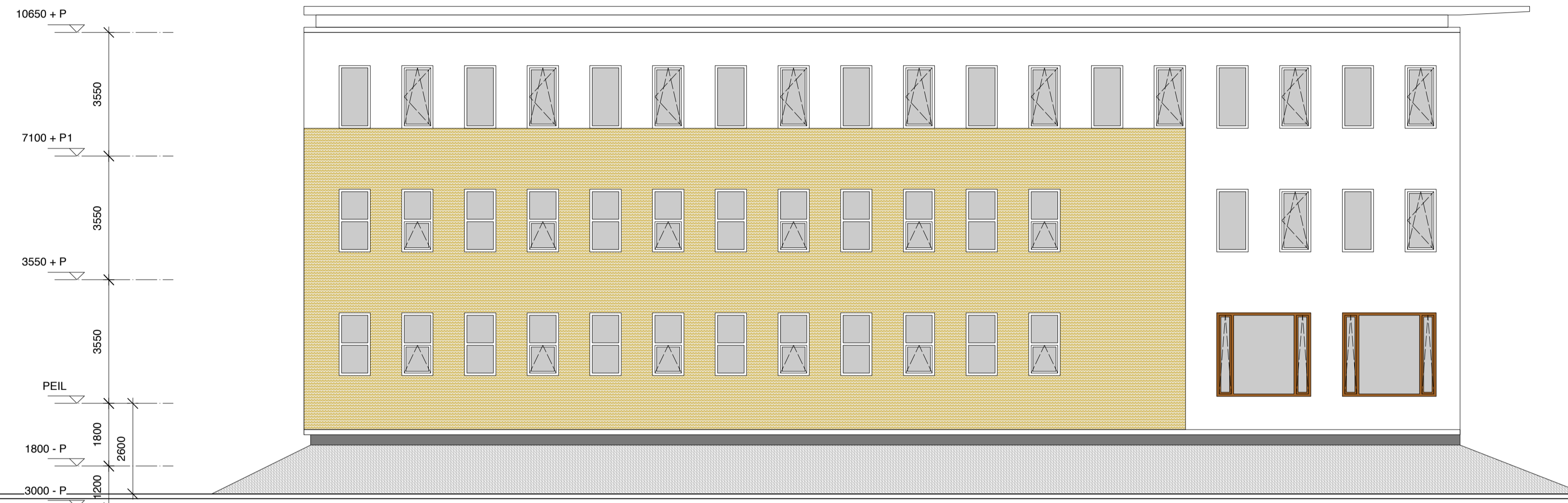
33160 GEVELAANZICHT VANUIT HET ZUIDEN 450 7200 7200 7200 7200 310 A B C D E F
