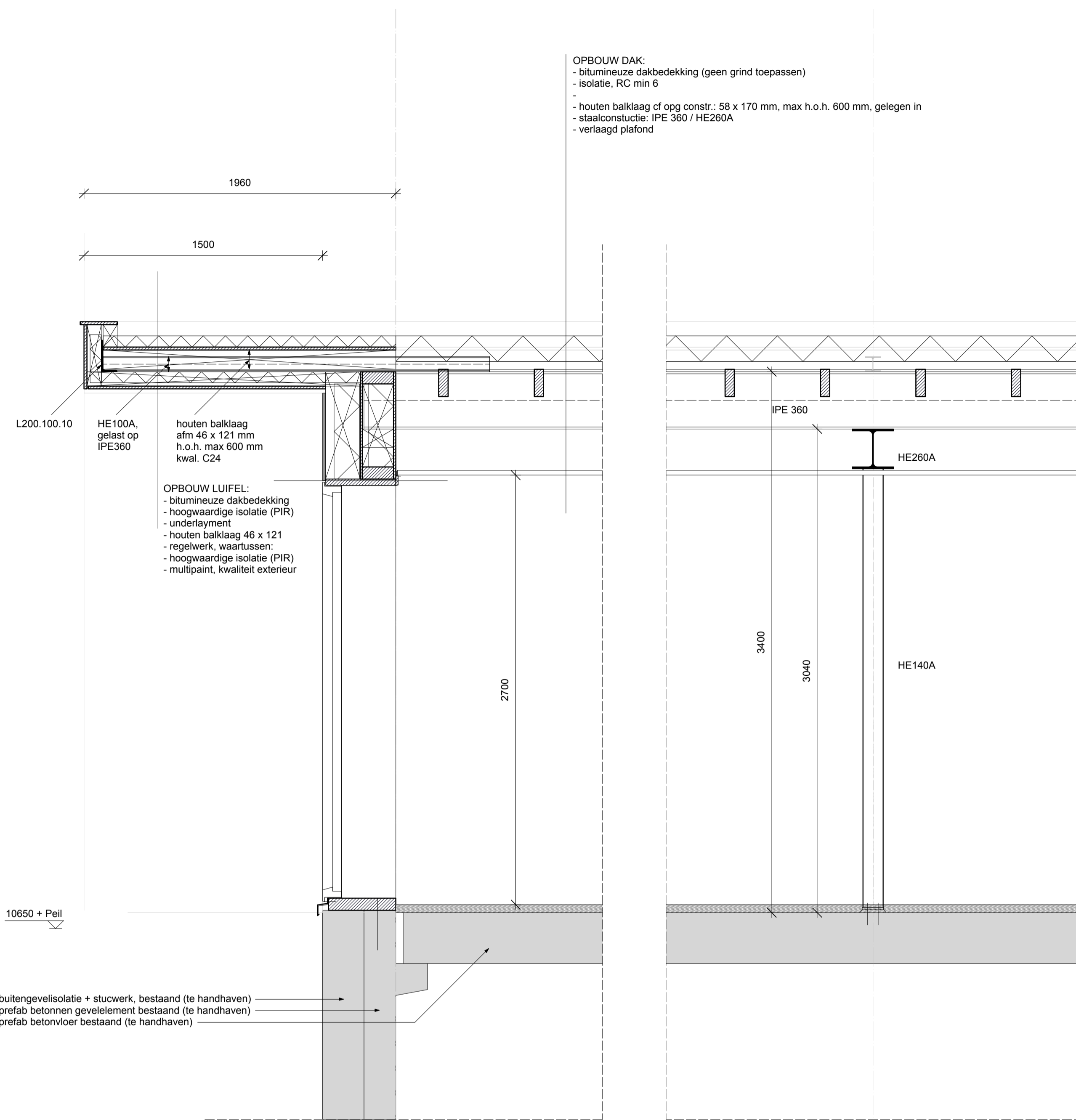
DOORSNEDE OVER ZIJGEVEL (DETAIL GELDT VOOR BEIDE ZIJGEVELS)
