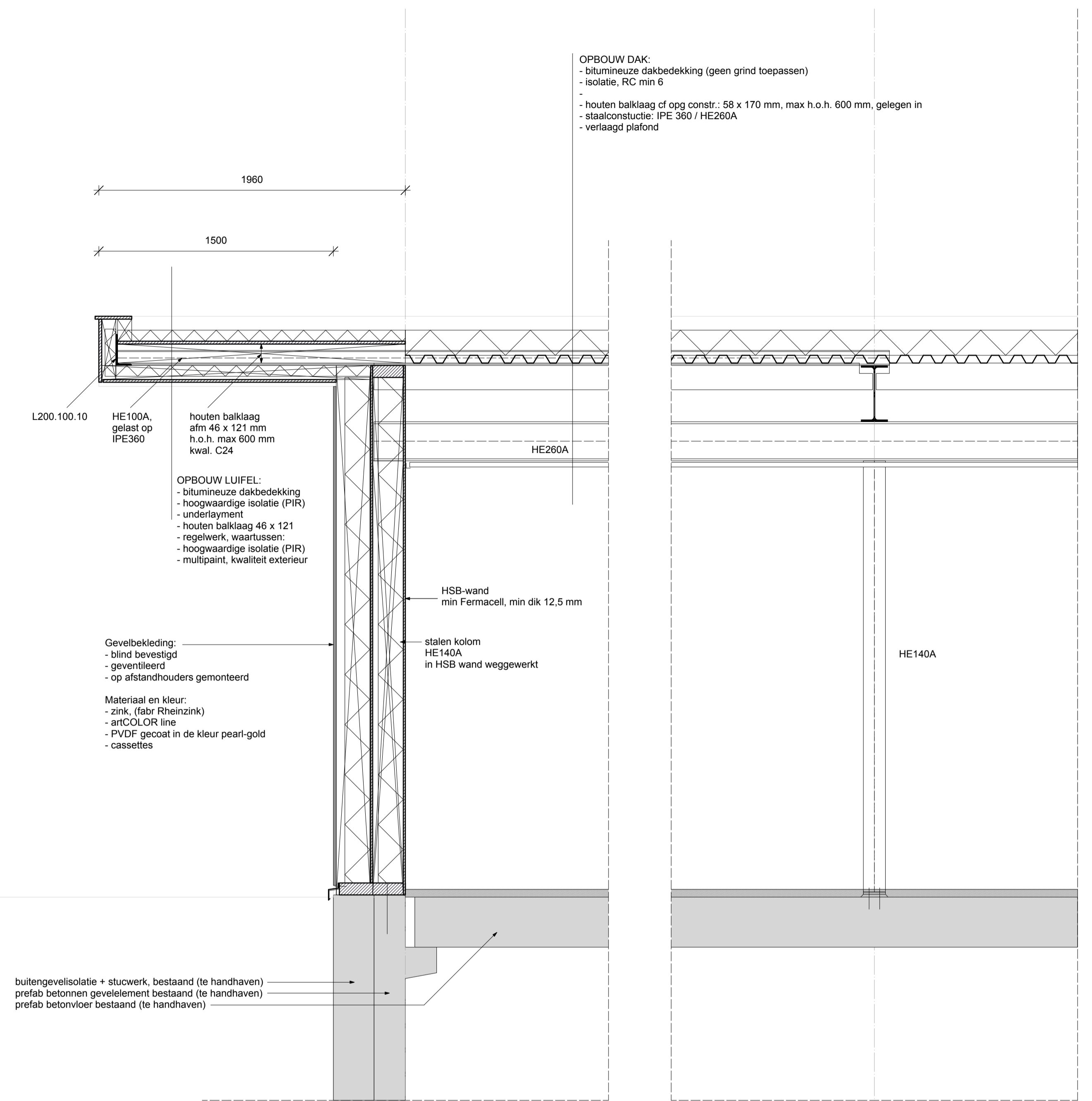
DOORSNEDE OVER GEVEL GELDT VOOR DE VOOR- EN ACHTERGEVEL
