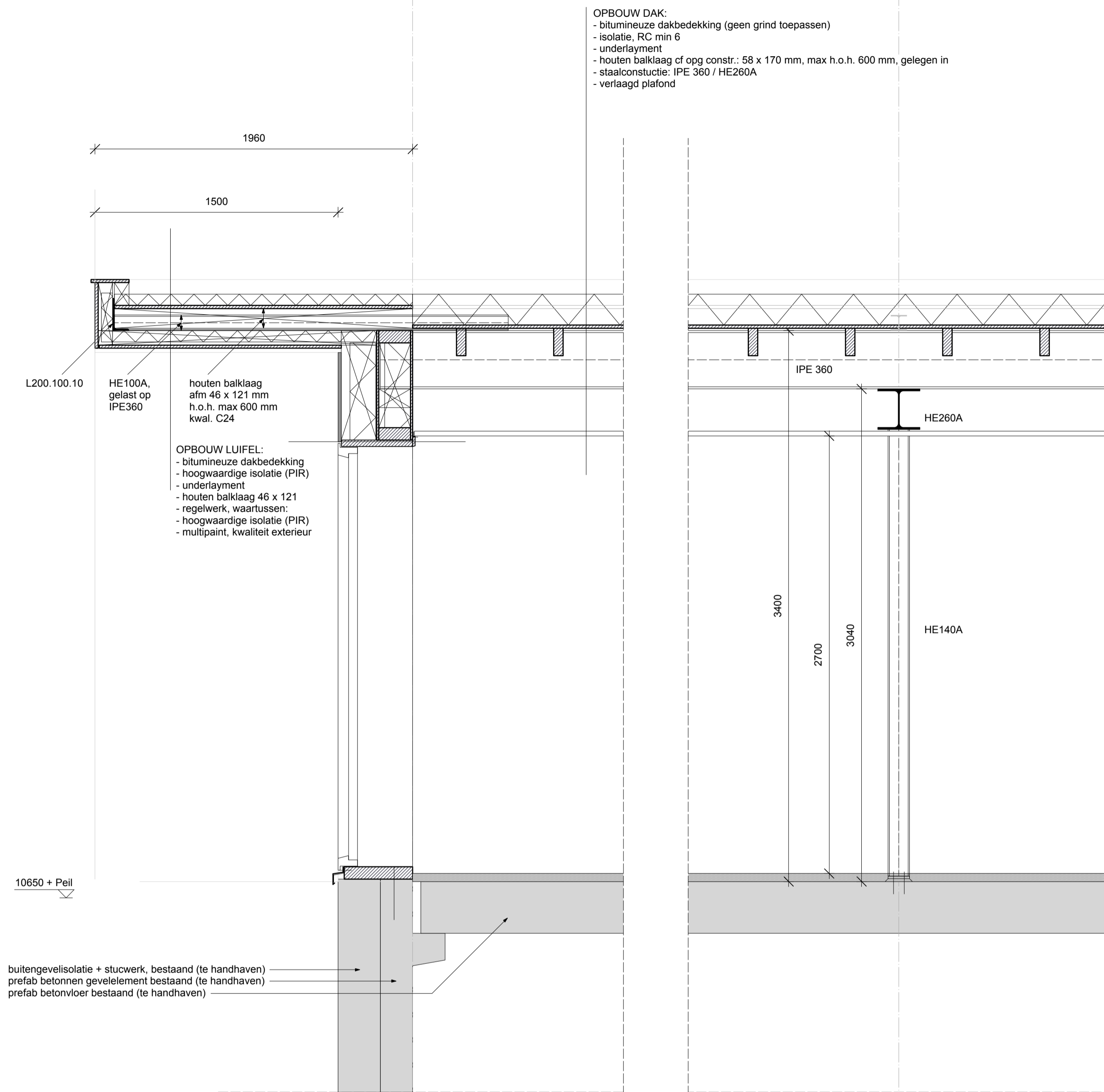
DOORSNEDE OVER ZIJGEVEL (DETAIL GELDT VOOR BEIDE ZIJGEVELS)
