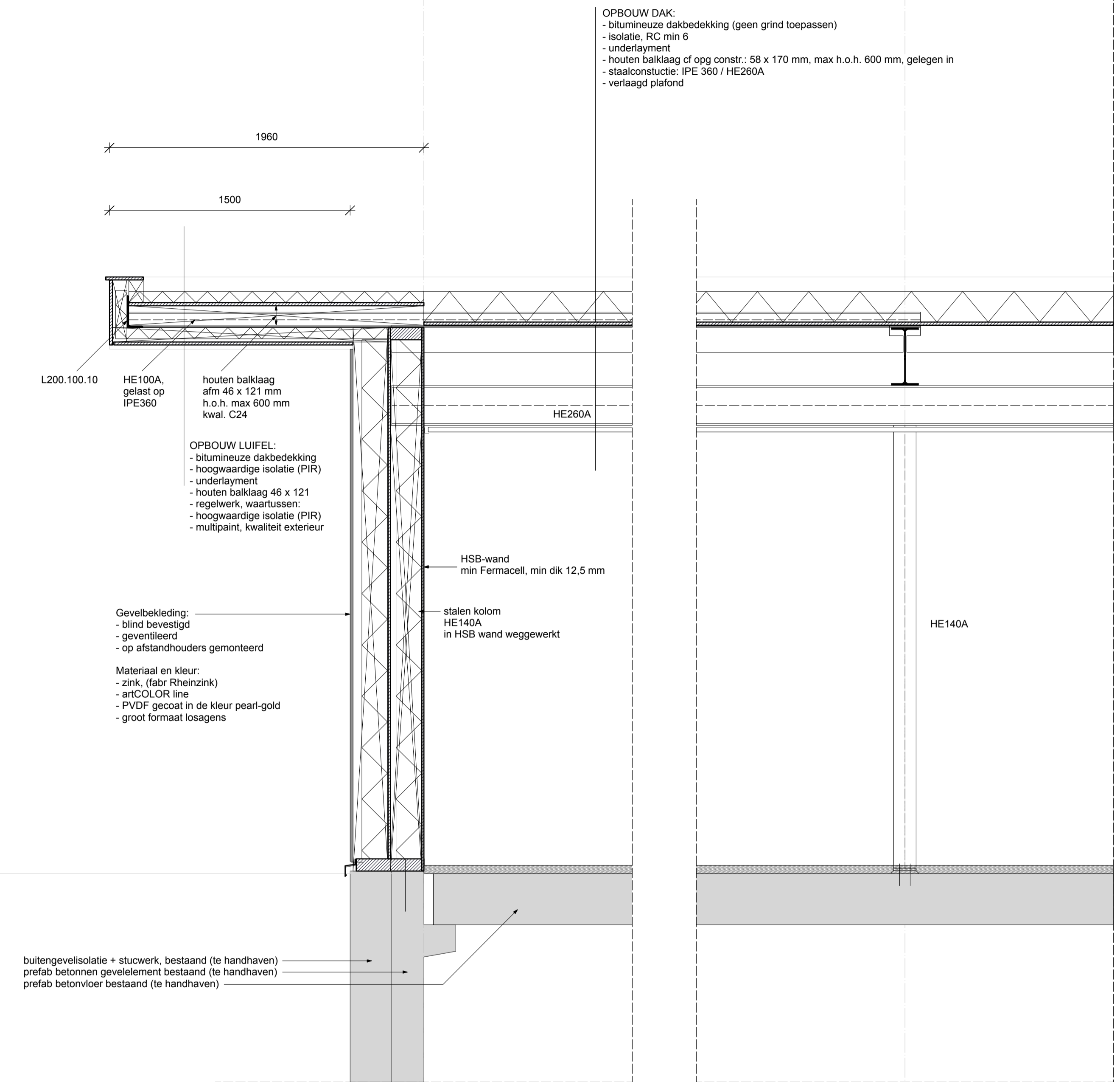
DOORSNEDE OVER GEVEL GELDT VOOR DE VOOR- EN ACHTERGEVEL
