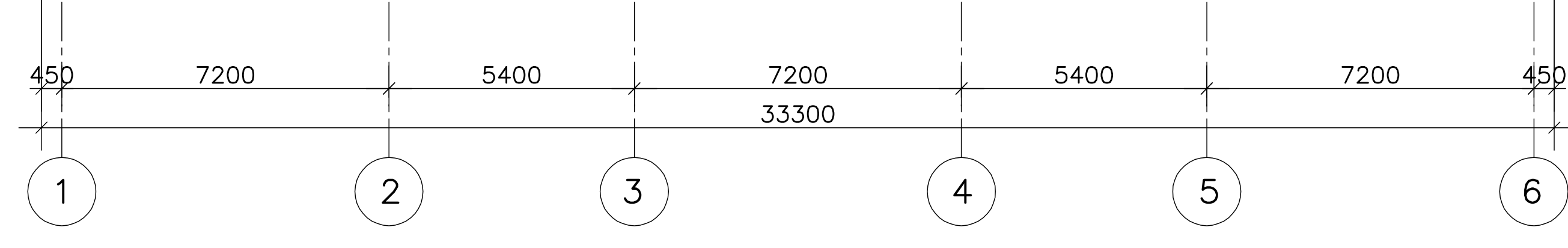
westgevel
