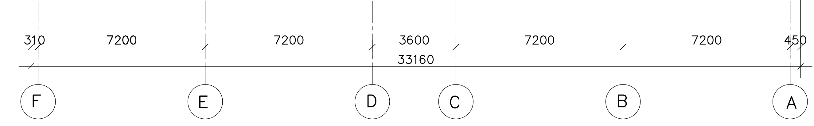
noordgevel
