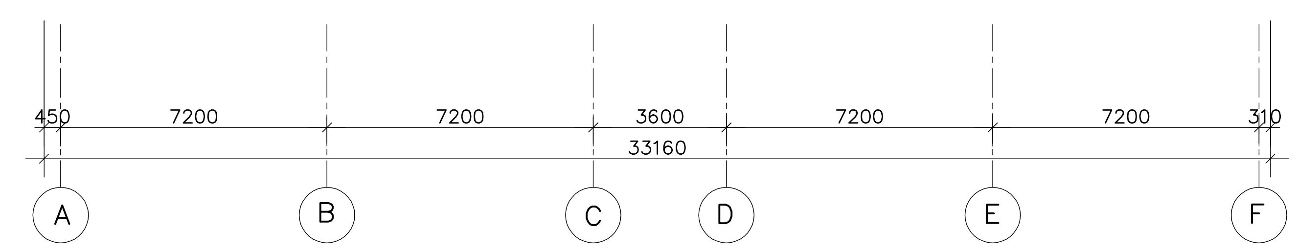
zuidgevel
